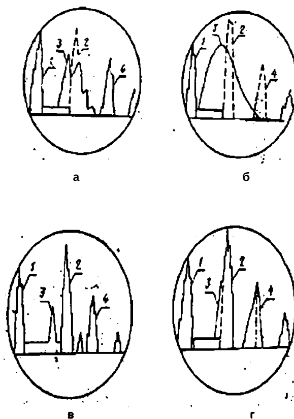
Рисунок В.1— Вид эхо-сигналов на экране дефектоскопа
